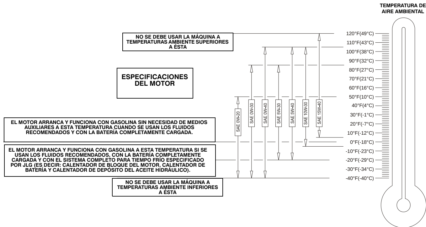
Figura 6-10. Especificaciones de temperaturas de funcionamiento del motor - Perkins - Hoja 1 de 2
