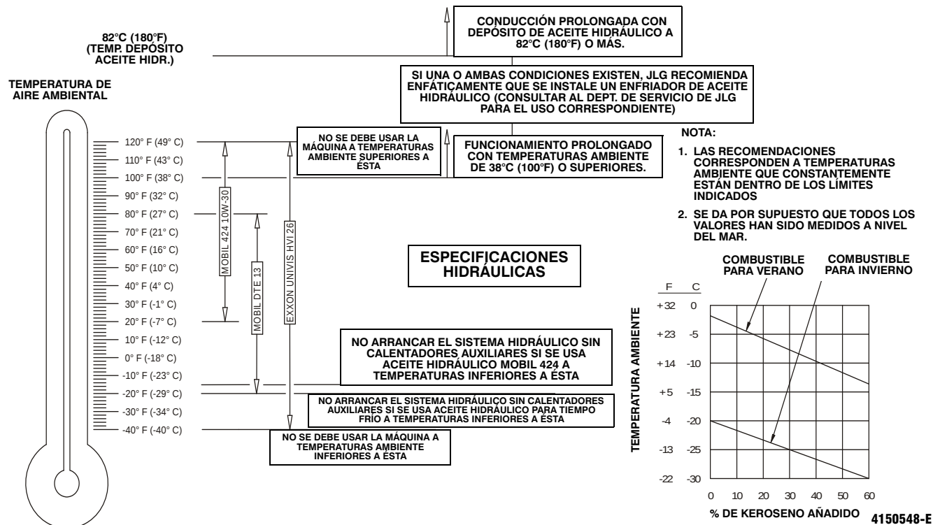
Figura 6-3. Especificaciones de temperaturas de funcionamiento del motor - Deutz - Hoja 2 de 2
