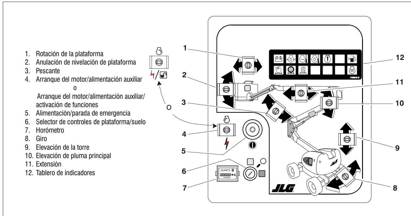
Figura 3-1. Estación de control del suelo - Modelos AJ
