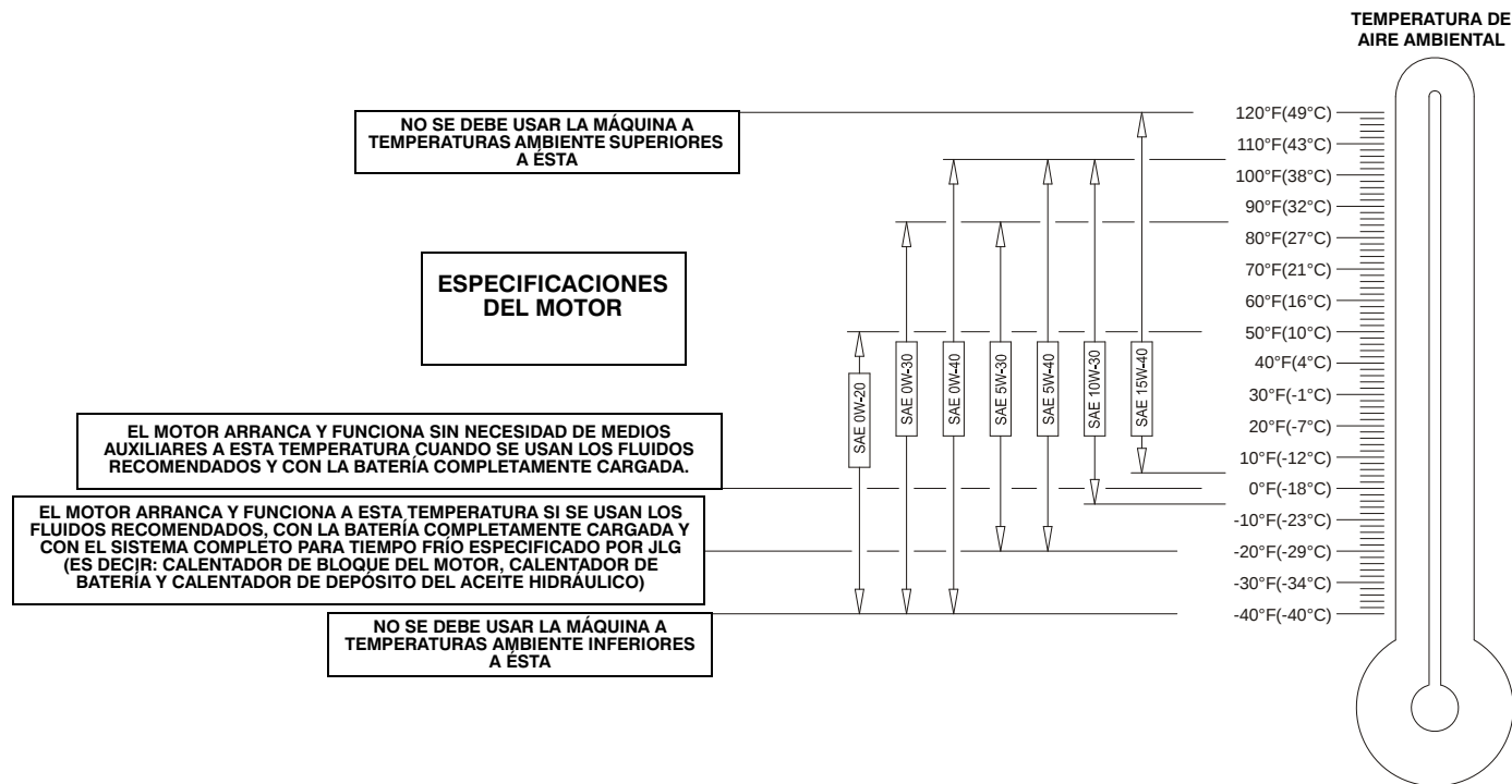
Figura 6-6. Especificaciones de temperaturas de funcionamiento del motor - Caterpillar - Hoja 1 de 2
